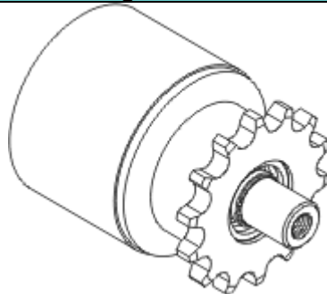
IGW = Achsende mit Einfachkettenrad und Innengewinde
