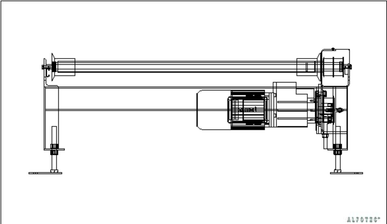
Prinzipskizze: Frontansicht
